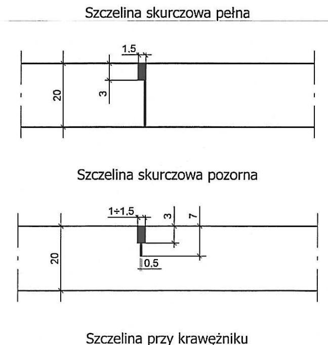
Rys. 1.1. Przykłady konstrukcji szczelin w podbudowie z betonu cementowego (wymiar w cm)
