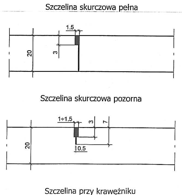
Rys. 1.1. Przykłady konstrukcji szczelin w podbudowie z betonu cementowego (wymiały w cm)
